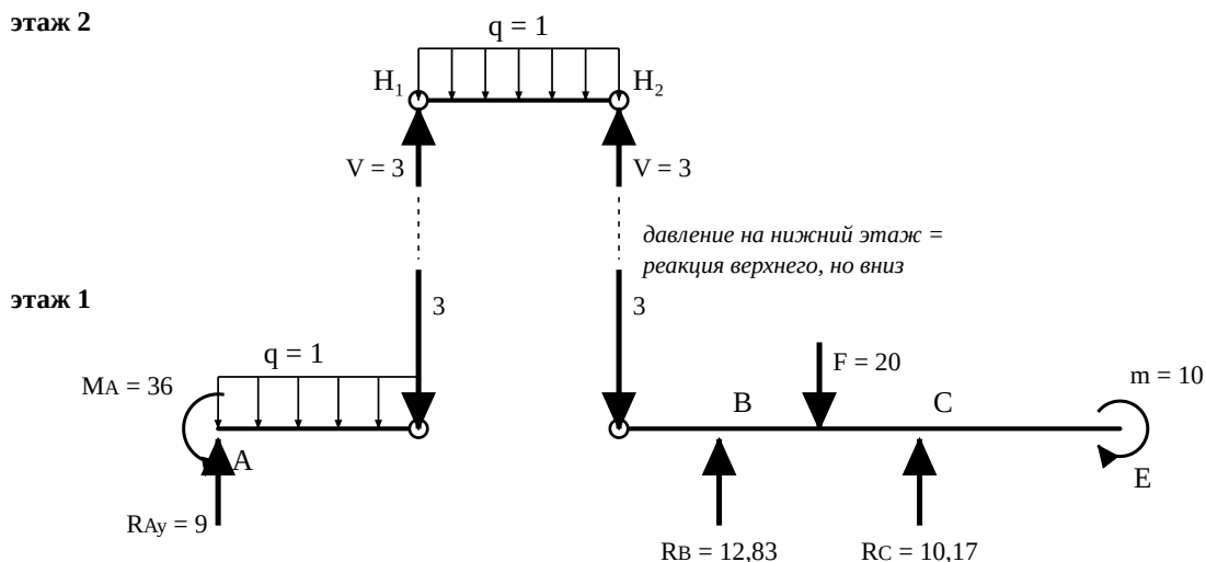
Схема 5 — этажи разнесены: реакции верхней балки Н 1 –Н 2 и её давление на нижние балки, опоры заменены найденными реакциями. Силы в кН, моменты в кН·м
