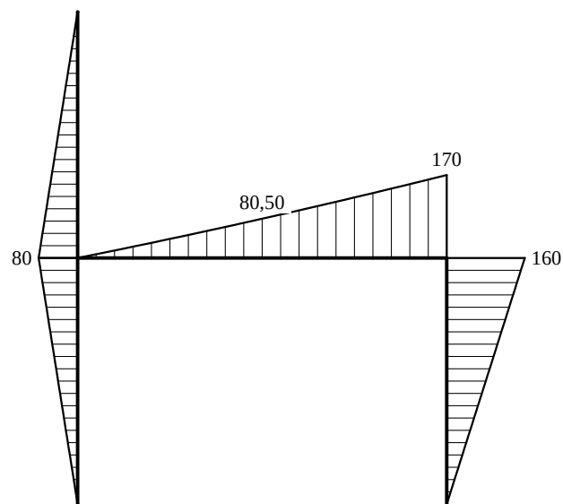
Схема 3 — эпюра M, кН·м
