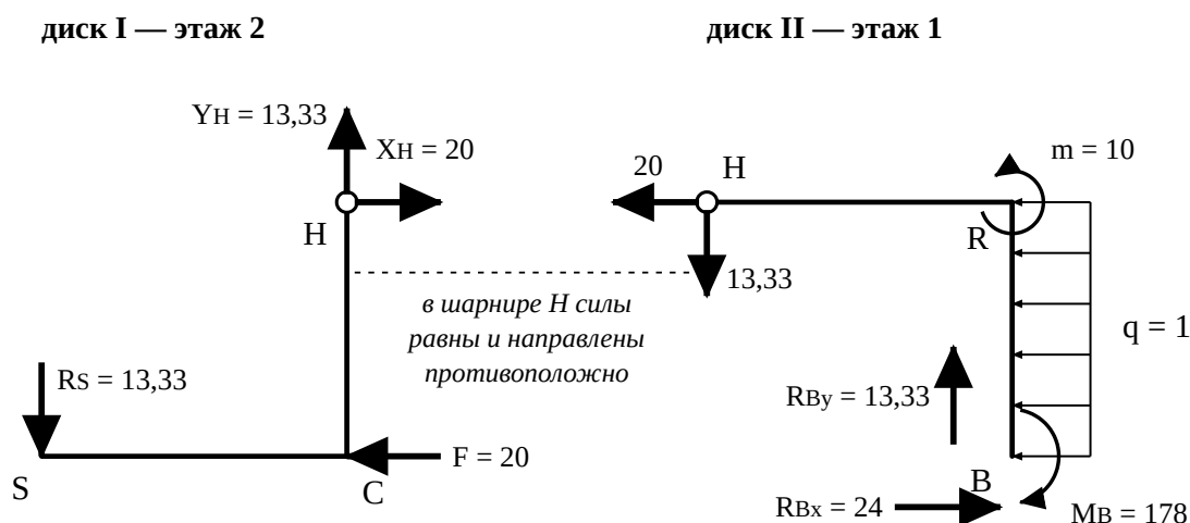
Схема 4 — этажи, разнесённые по шарниру H: найденные реакции в истинном направлении и давление диска I на диск II. Силы в кН, моменты в кН·м
