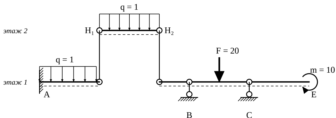
Схема 5 — поэтажная схема. Пунктир — отмеченное (нижнее) волокно. Силы в кН, моменты в кН·м
