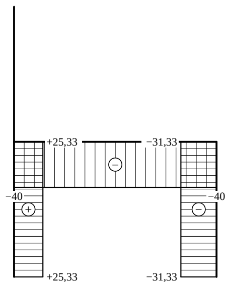
Схема 3 — эпюра N, кН
